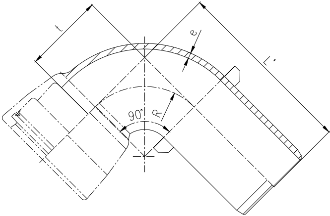
图11 承插90° 弯头
