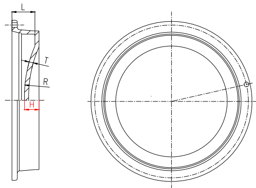
图 38 DN>300 K 型插堵
