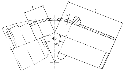
图12 承插45° 弯头
