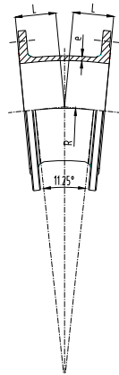
图19 双盘11.25° 弯头
