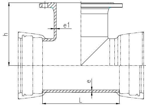
图 25 双承单支盘三通
