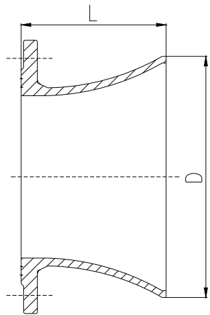
图 48 喇叭口
