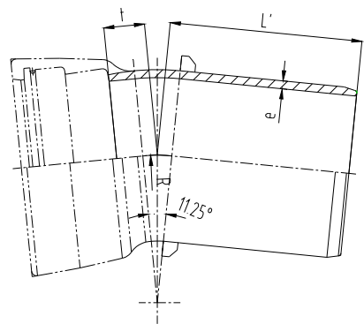
图14 承插11.25° 弯头
