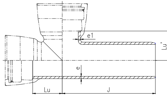
图 28 承插单支承三通
