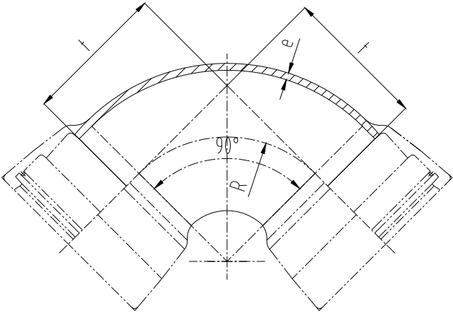
图7 双承90° 弯头
