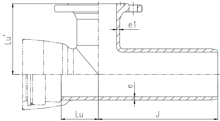
图 29 承插单支盘三通
