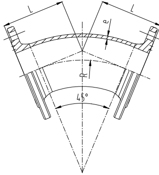
图17 双盘45° 弯头
