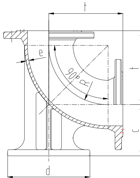
图 20 双盘 90° 鸭掌弯头
