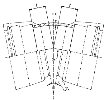
图9 双承22.5° 弯头
