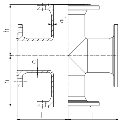
图 35 全盘四通
