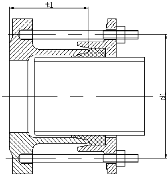
图 46 法兰接头
