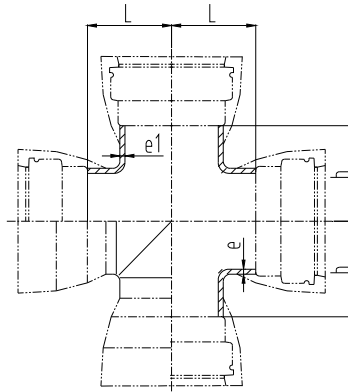
图 34 全承四通
