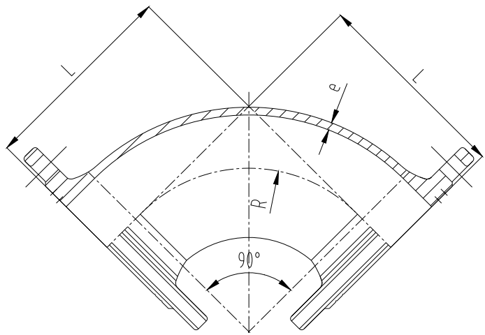
图16 双盘90° 弯头
