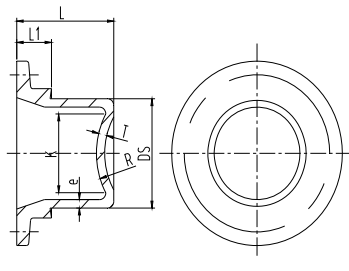
图 42 DN>300 K 型承堵
