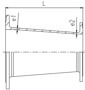
图 22 双盘渐缩管
