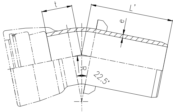
图13 承插22.5° 弯头
