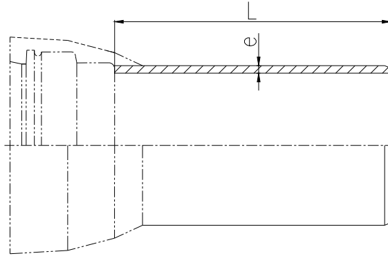
图2 承插
