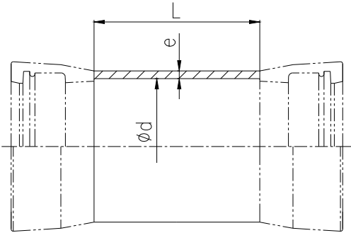
图3 T型承套
