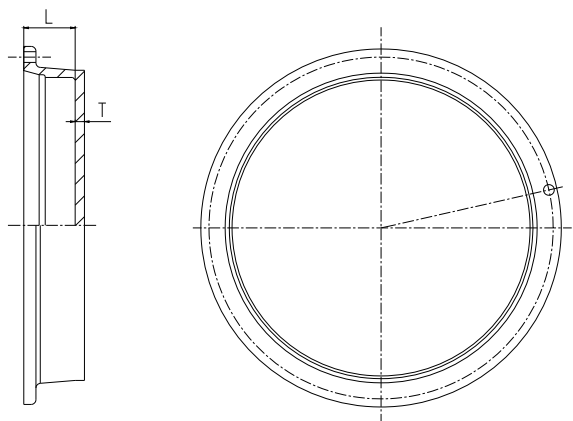
图 37 DN≤300 K 型插堵
