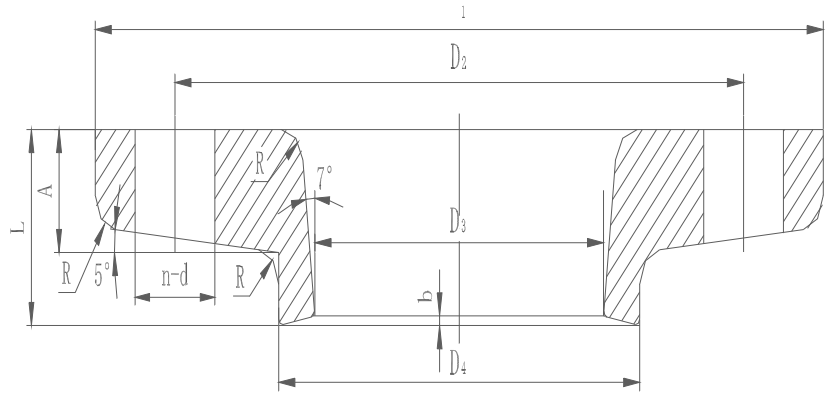
图 55 K 型接口压兰
