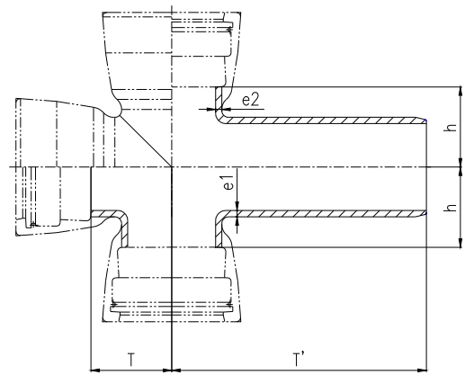
图 36 承插双承四通 表 37 承插双承四通的尺寸和重量
