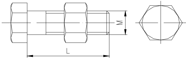
图 57 法兰盘连接用螺栓
