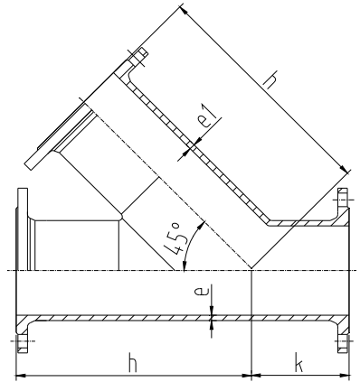
图33 全盘45° 斜三通
