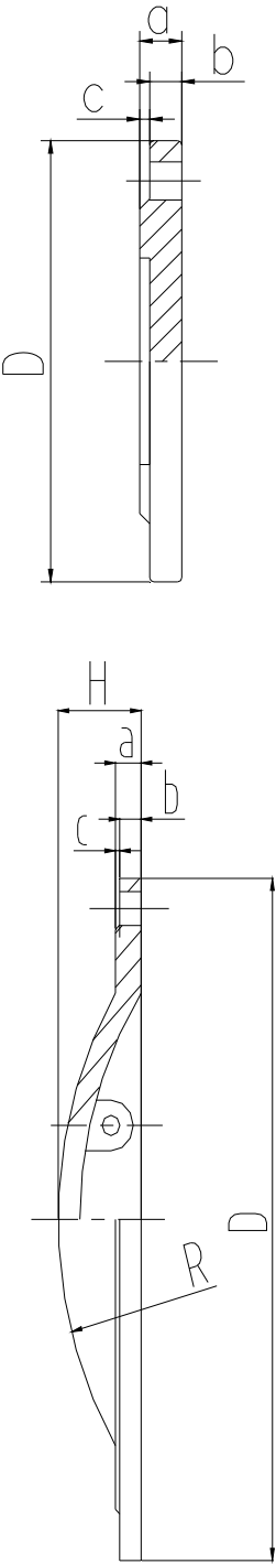
图52 法兰盲板
