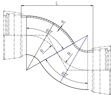
图 23 双承乙字管
