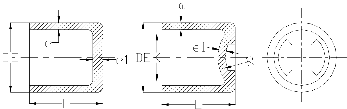
图43 T型承堵
