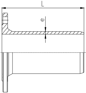
图1 盘插
