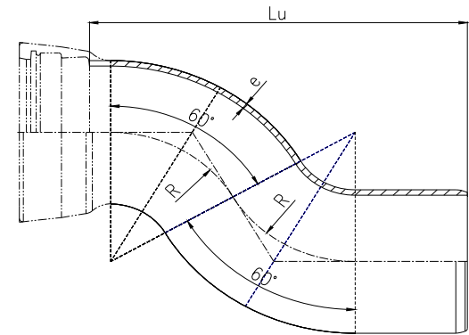
图24 承插乙字管
