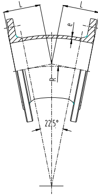
图18 双盘22.5° 弯头
