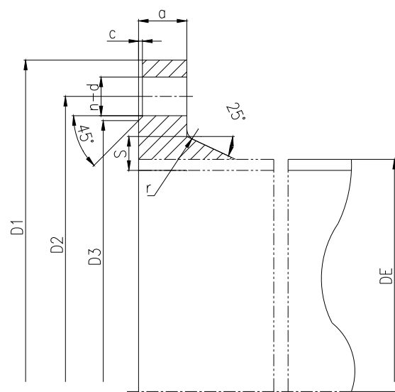
图49 法兰盘
