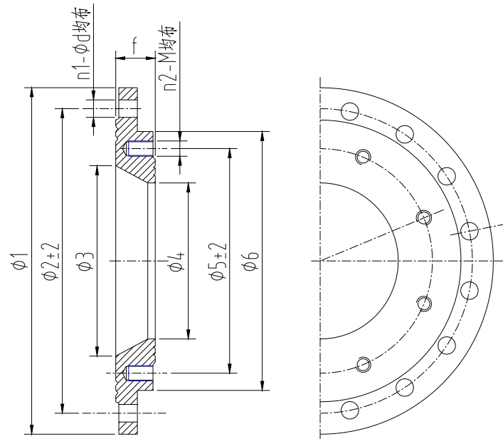
图 52 减径法兰
