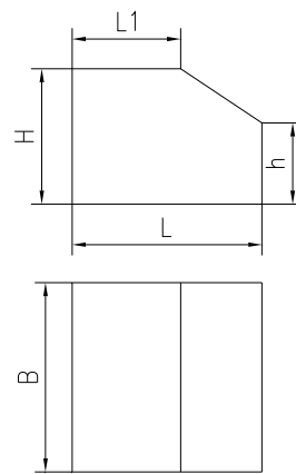
图 15 安装块
