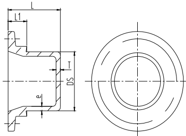
图 41 DN≤300 K 型承堵
