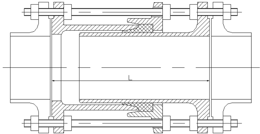
图 47 可拆卸接头
