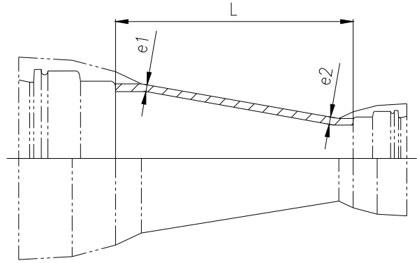
图 21 双承渐缩管
