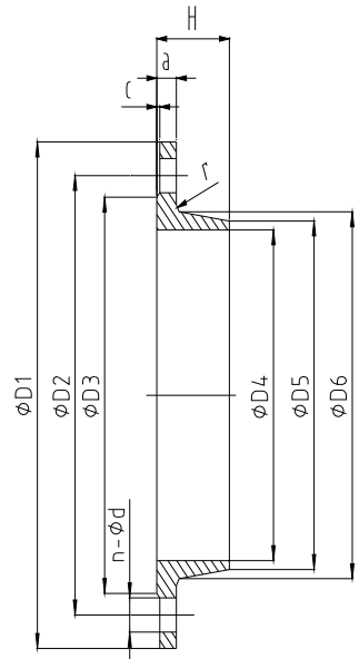
图50 焊接法兰
