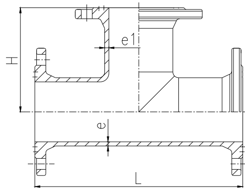
图26 全盘三通
