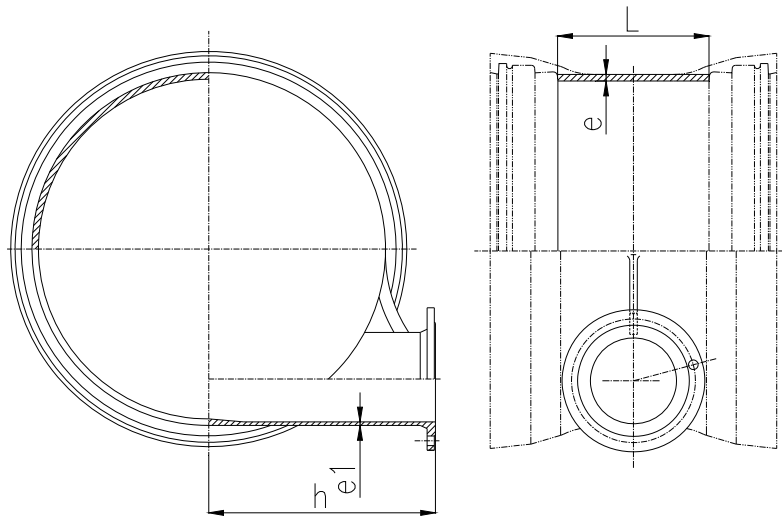
图30 双承单支盘底三通
