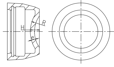
图40 DN>300 T型插堵
