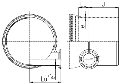
图 44 承插单支盘底三通
