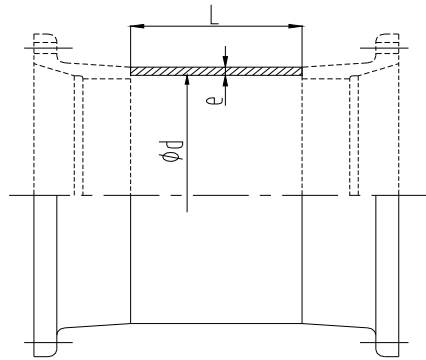
图4 K型承套
