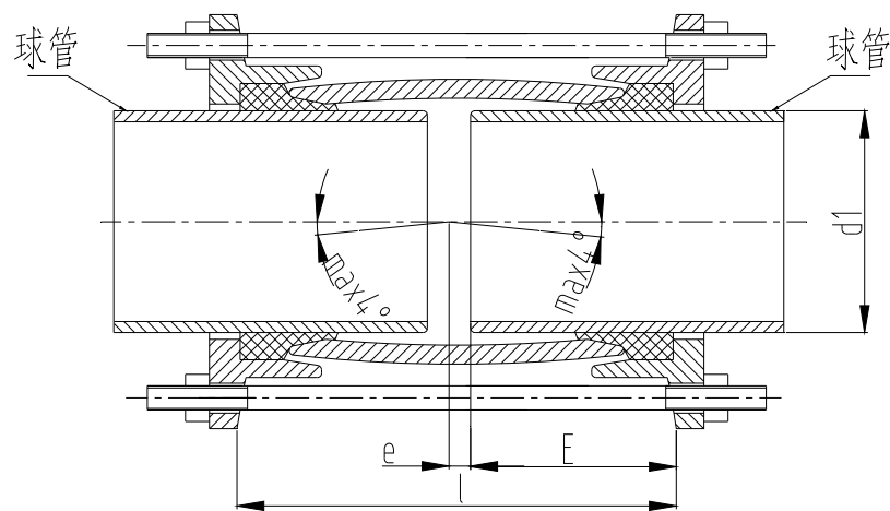
图 45 柔性接头
