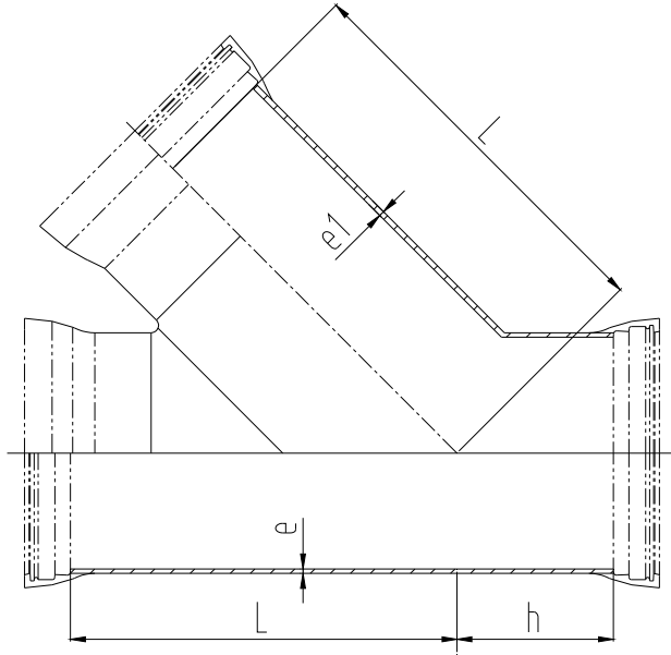
图 32 全承 45° 斜三通
