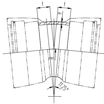
图10 双承11.25° 弯头
