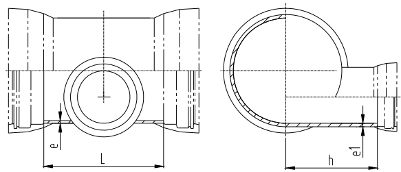
图 31 全承底三通
