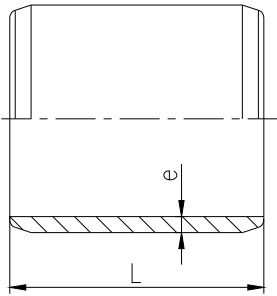
图6 双插
