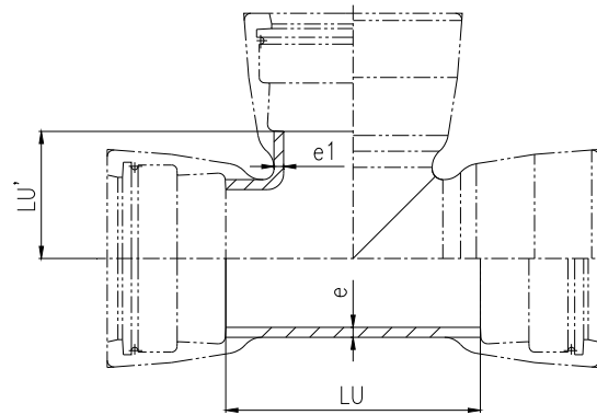
图 27 全承三通
