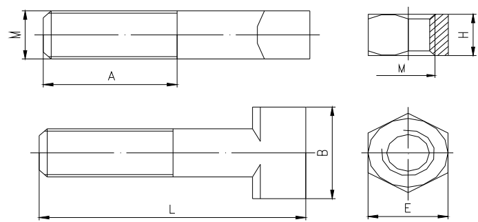
图56 K型接口用螺栓
