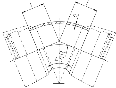
图8 双承45° 弯头
